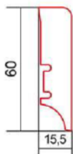
P6P Profil
