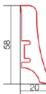
P 20 Profil
