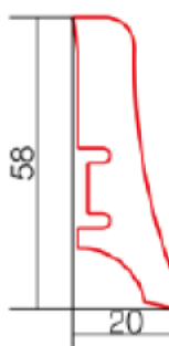
P 20 Profil
