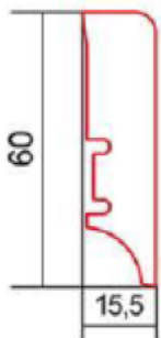
P6P Profil
